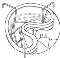
Demontage des Filterschlauchs mit Snap-Ring
