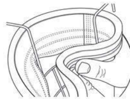
Montage des Filterschlauchs mit Snap-Ring
