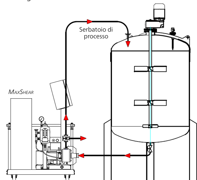
Schema di processo MAXSHEAR
