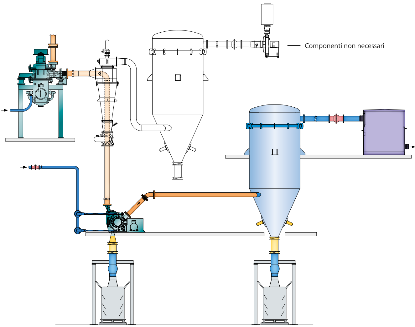
Impianto di macinazione e classificazione con INLINESTAR e jet mill CGS montato a monte, in esecuzione resistente allo scoppio
