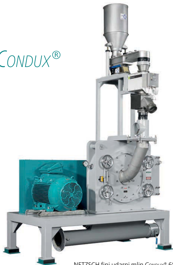
NETZSCH fini udarni mlin CONDUX® 680
