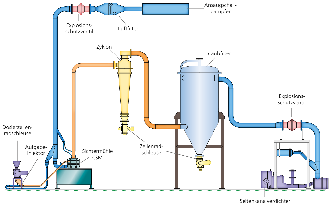
Druckstoßfeste Mahlanlage
