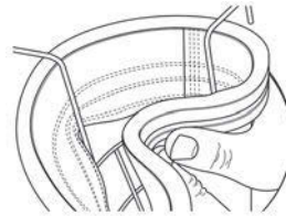
Montaggio della manica tramite anello filtrante
