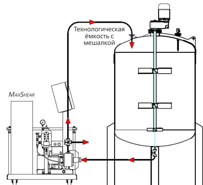
Схема технологического процесса на MaxSHEAR
